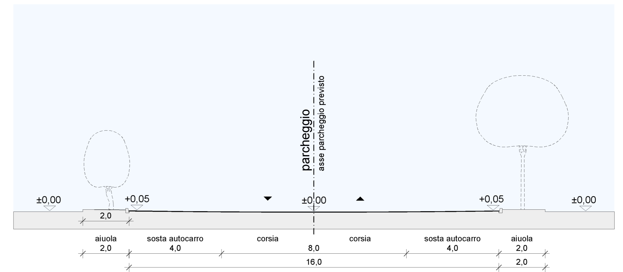
SEZIONE F - F
