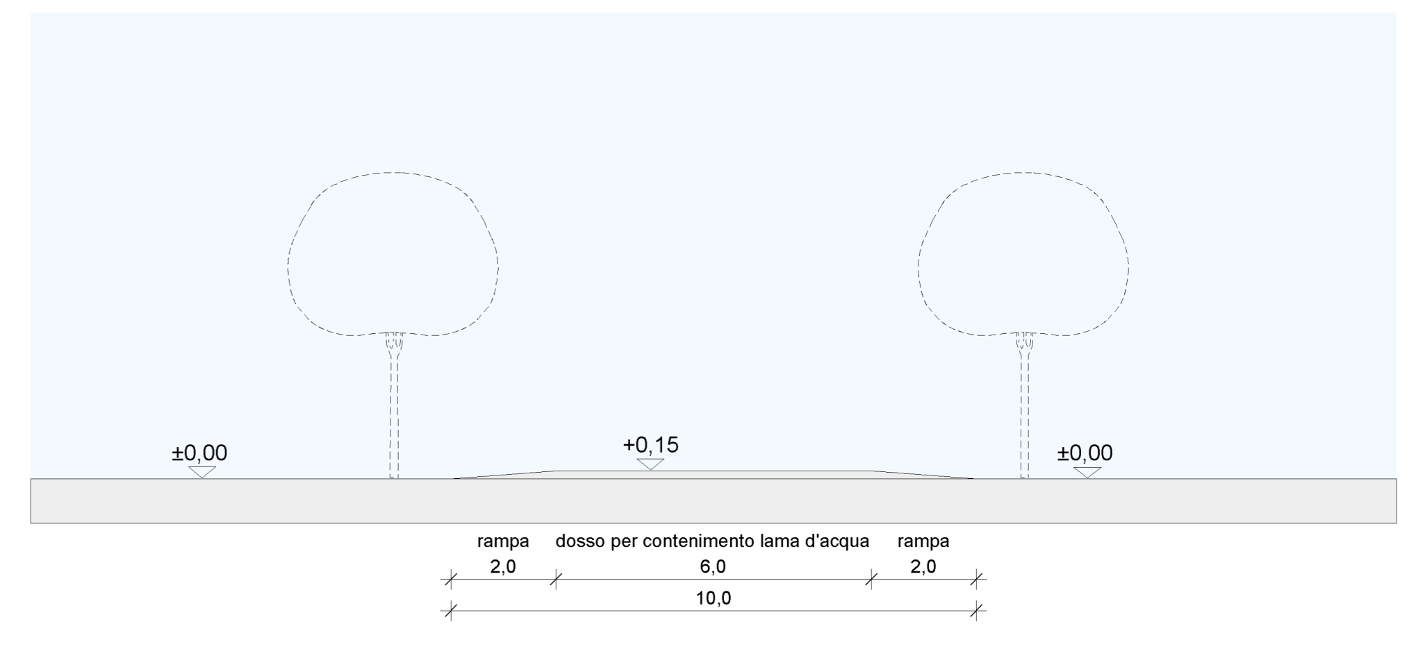
SEZIONE H - H
