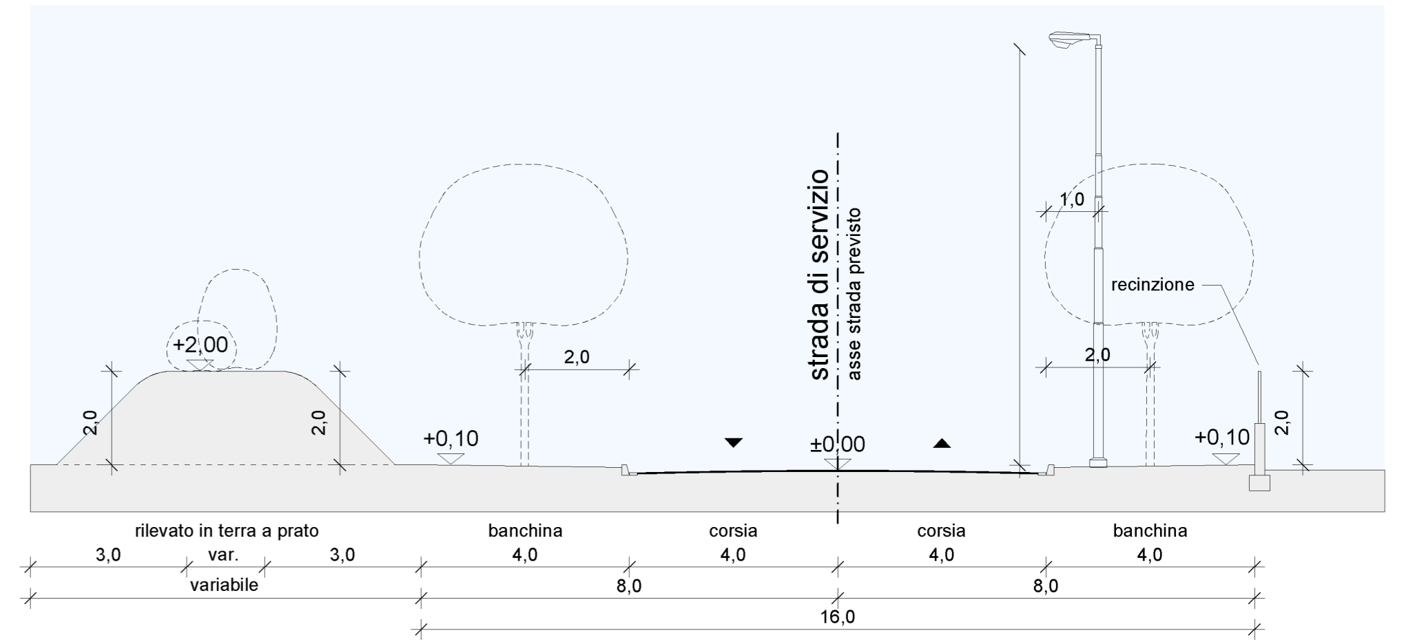
SEZIONE D - D
