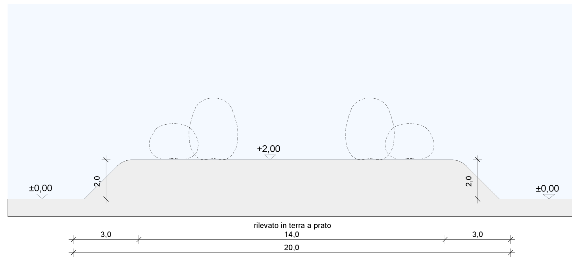
SEZIONE E - E
