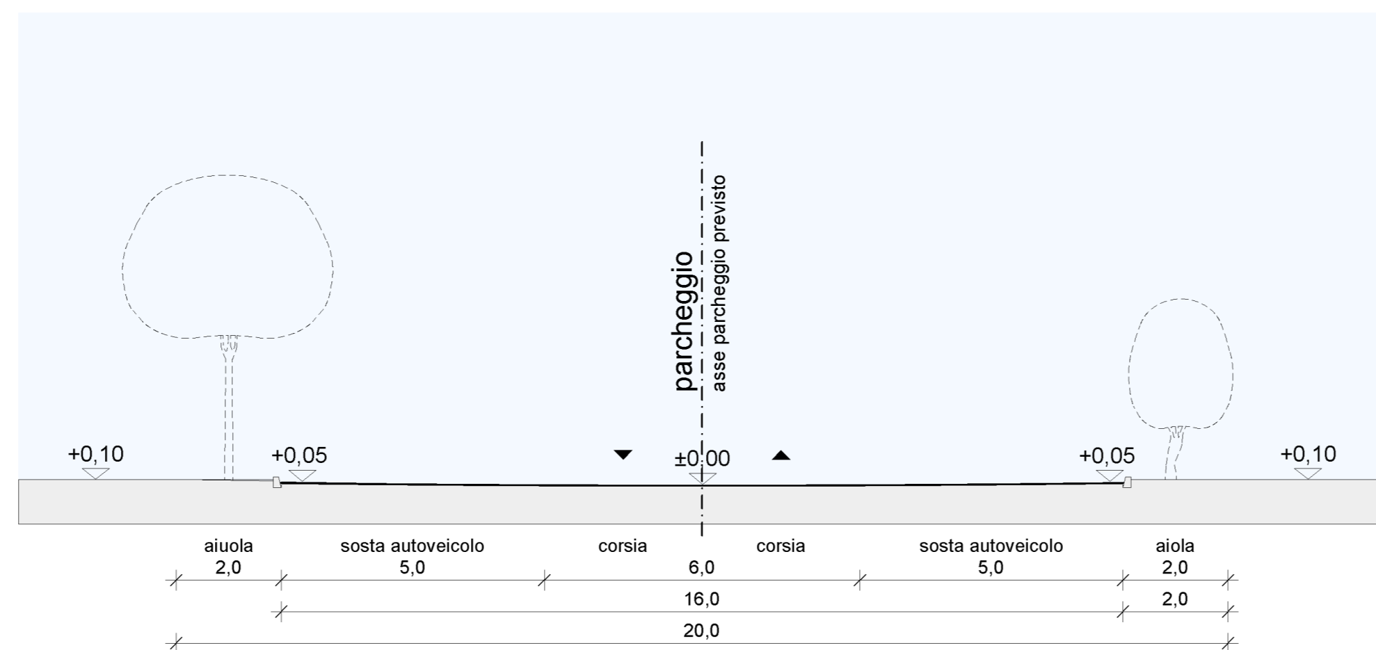
SEZIONE G - G
