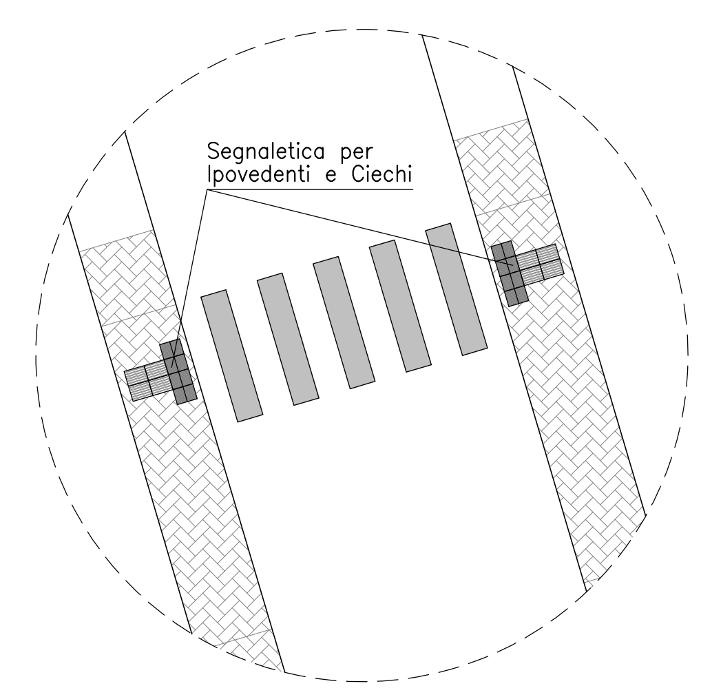
PARTICOLARE ATTRAVERSAMENTO Scala 1:100
