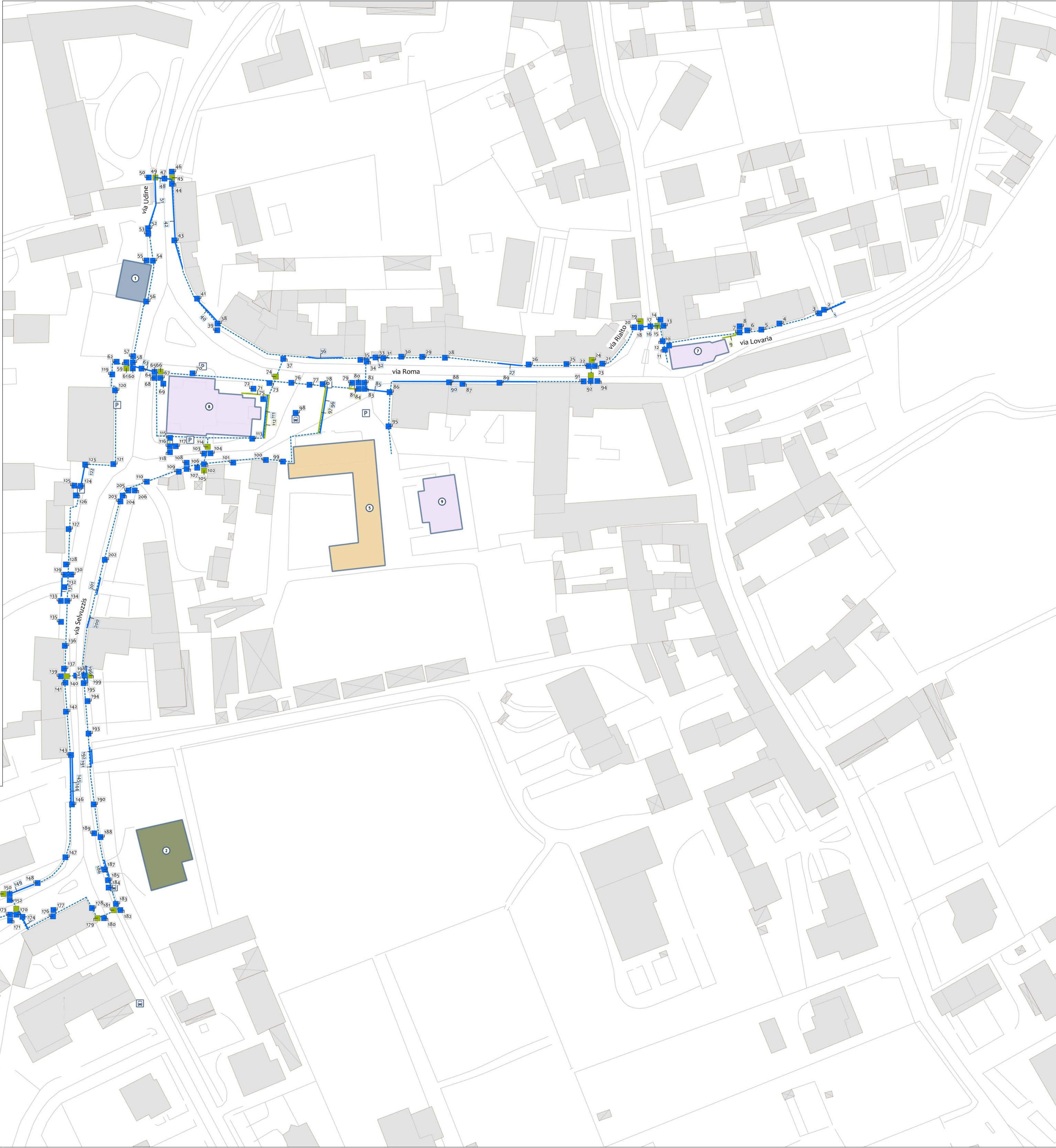
PLANIMETRIA_PAVIA DI UDINE scala 1:750
