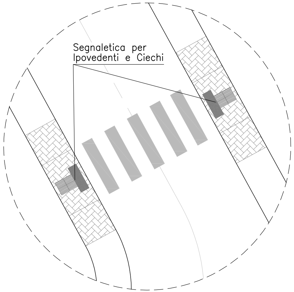
PARTICOLARE ATTRAVERSAMENTO Scala 1:100
